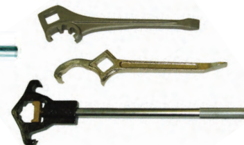
Clés de manipulation (divers modèles)
