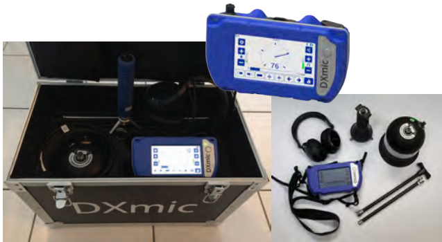
Détecteur acoustique DXMIC
